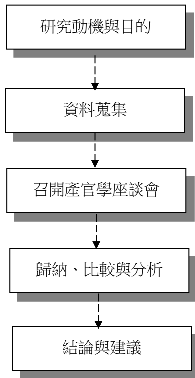
圖 1-1：研究流程圖
